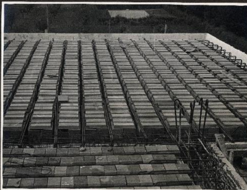
Copertura in cemento armato del salone di ricevimento
