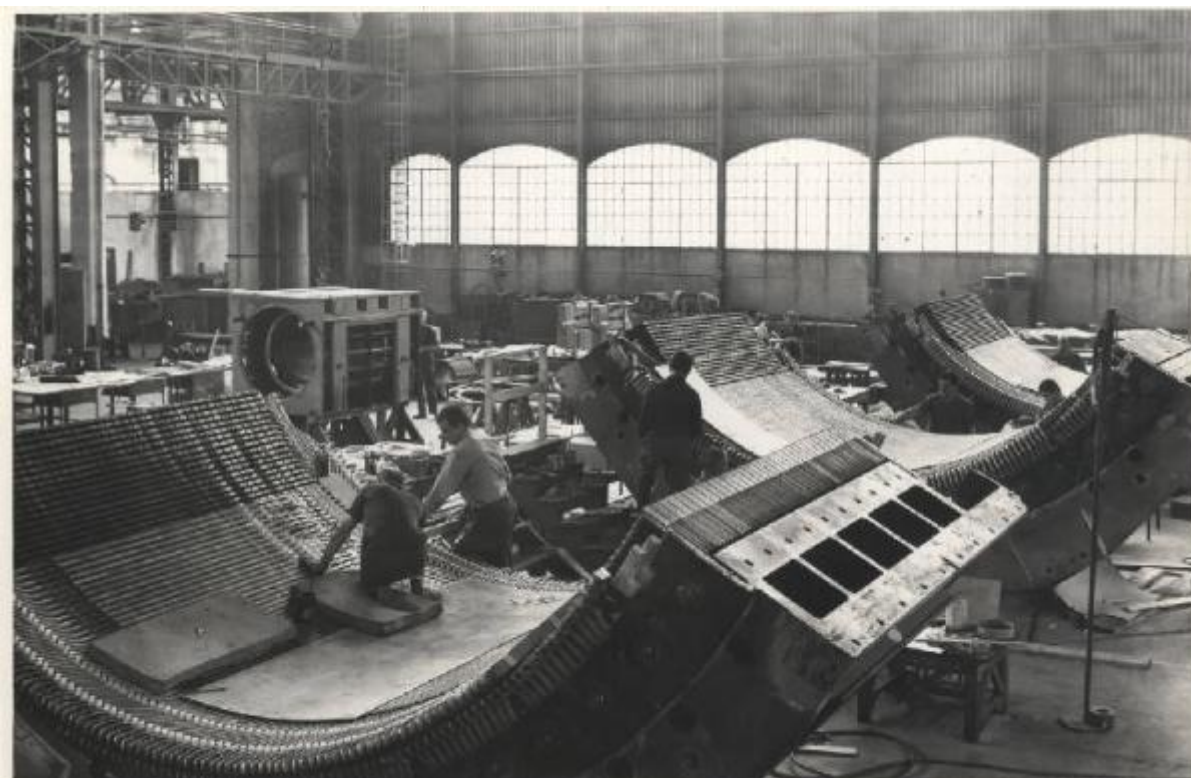
10256/957 - 2 alternatori 90.000 kVA - 11.800+10%-5% V - 50 Hz - 333,3 giri/1' Messa in opera delle sbarre statore per E.N.E.L. - ROMA - Centrale di Monte S. Angelo
