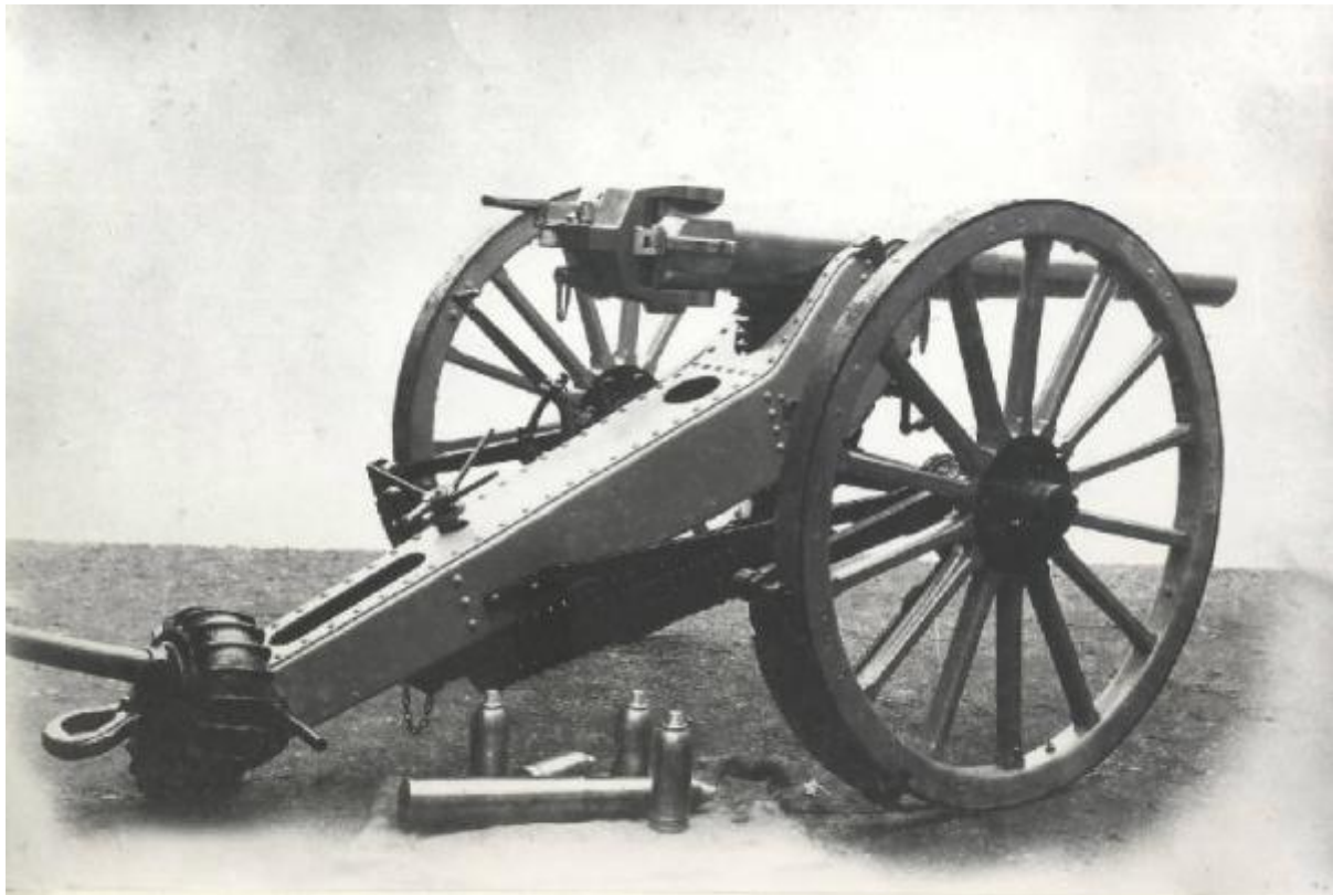
Primo cannone da campagna - Calibro 75 - costruito dalla Società Ing. ERNESTO BREDÀ e C. nel 1897
