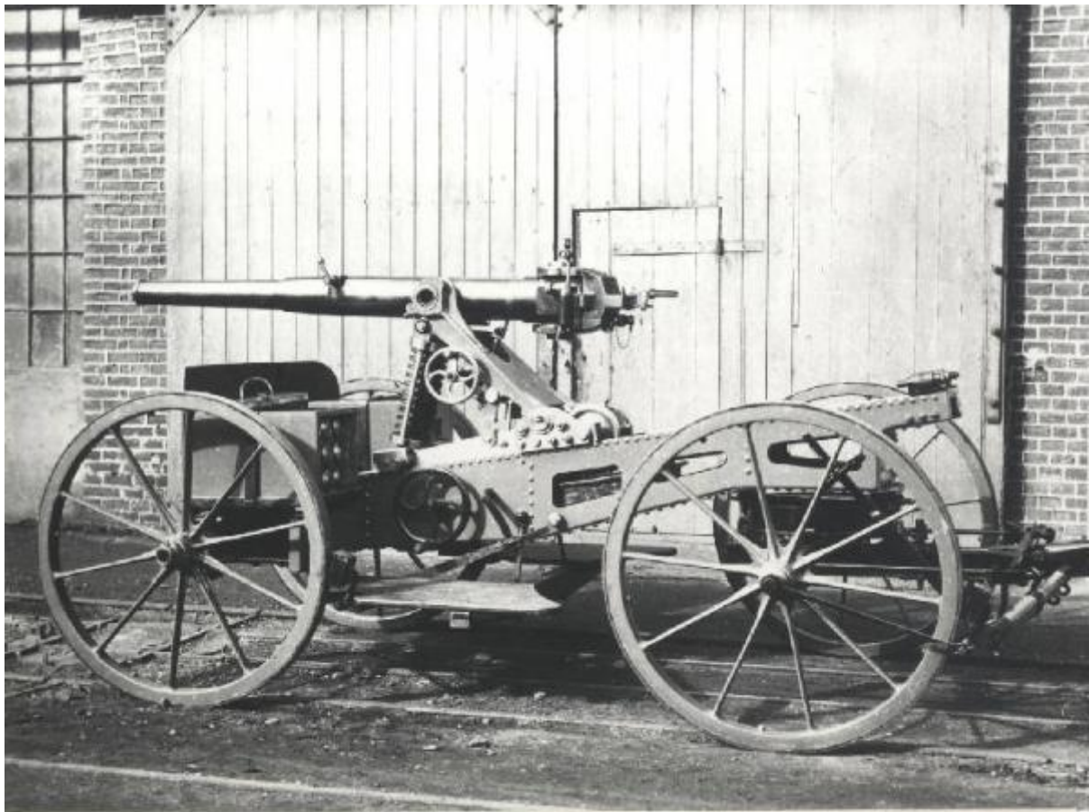
Primo cannone da campagna - Calibro 78 - costruito dalla Società Ing. ERNESTO BREDA e C. nel 1897
