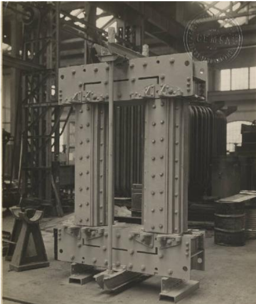
SOCIETA' PER COSTRUZIONI ELETTROMECCANICHE DI SARONNO "C. E. M. S. A." Nucleo del trasformatore monofase a raffreddamento naturale in olio 1500 KVA. - 59.300/4200 Volta - 16 \frac{2}{3} periodi ("F. S." - BOLZANO - BRENNERO) (L. 10 1-1928)
