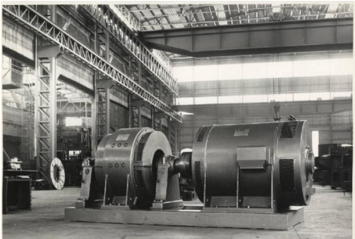
1965 - n.2 gruppi convertitori Motore asincrono trifase 750 HP - 3000 V - 50 Hz - 980 g/1' Dinamo 500 kW - 500 V - 1000 A - 980 g/1' per Soc. A.L.C.E. - Roma
