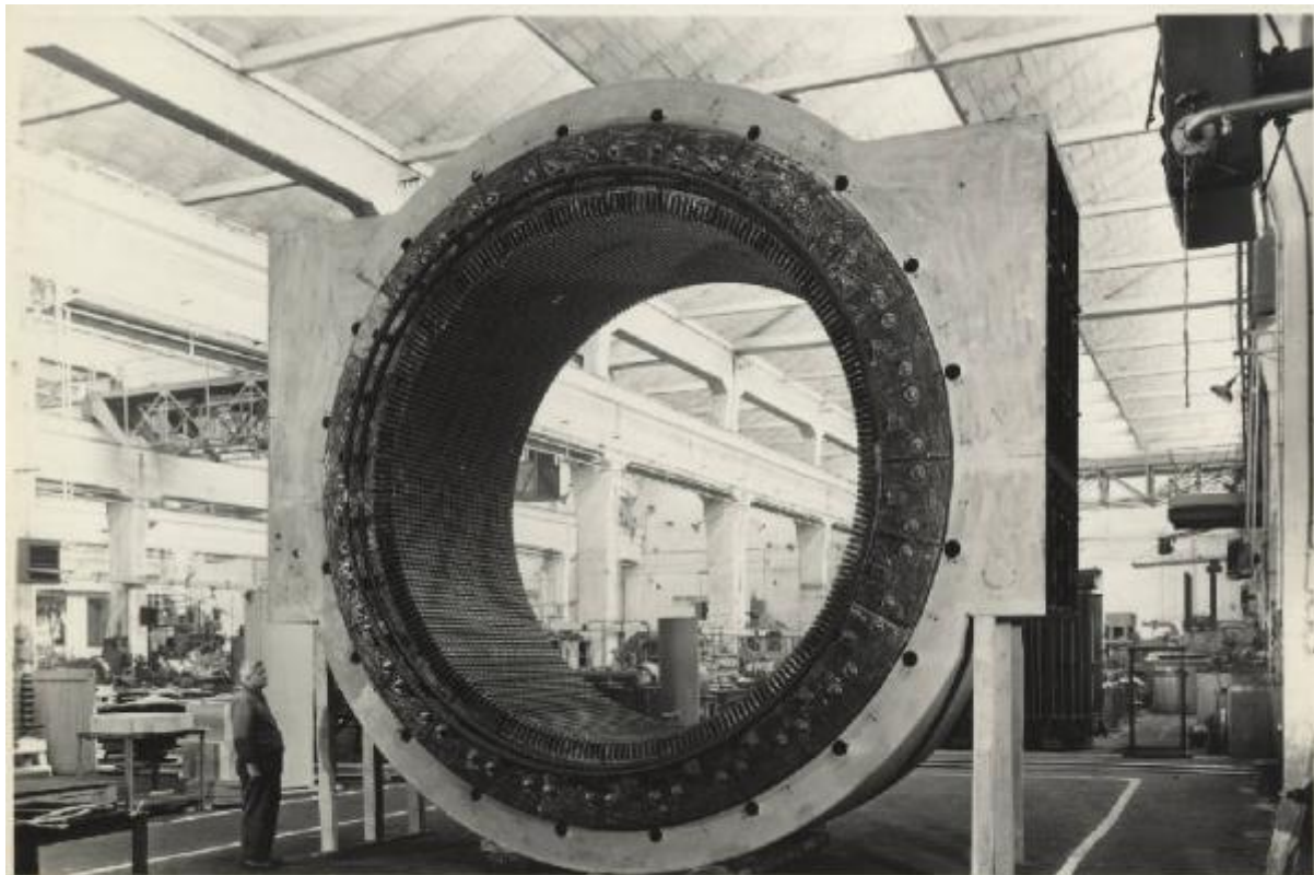
1960 - 2 Generatori - Motori sincroni trifasi 43500 kVA - 10000 V.-50 Hz-428 giri/1' per Soc. Generale Elettrica della Sicilia - C.le di Guadalupe Statore composto con anelli ancoraggio, prima del montaggio avvolgimenti
