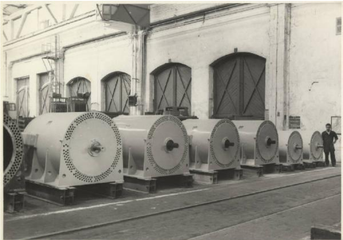
1962 - 6 Motori trifasi asincroni da 230+900 HP - 6000 V - 50 Hz - 590+1490 giri/1' per Società Tifec - C.le di Ternini Incease
