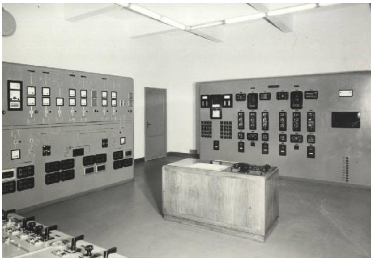
1949 - Quadro di comando e manovra per Società Idroelettrica Piemonte - C.la di Pontey
