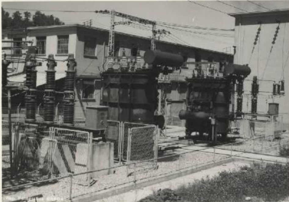
28. Anno 1944 - Cartiera vite Mayer - Stabilimento di Ceirate 2 trasformatori trifasi 10.000 kVA - 44,5/11+6,35 kV - 50 Hz
