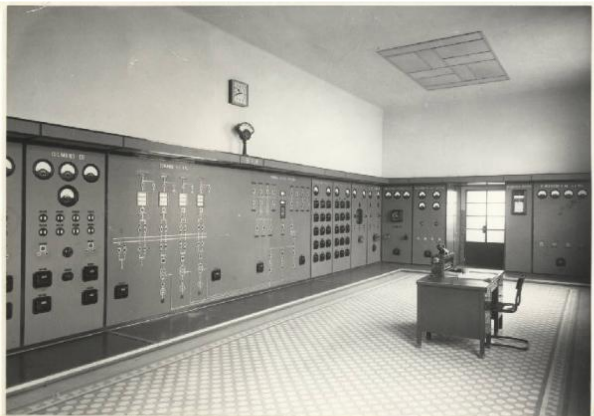
1930 - Quadro per sottostazione di conversione per Ferrovie Italiane dello Stato
