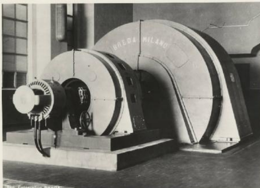
15. Anno 1941 - Società Idroelettrica Piemonte - Cabina Torretta Condensatore sinorono 15.000 kVA - 13 kV - 750 giri - 50 Hz
