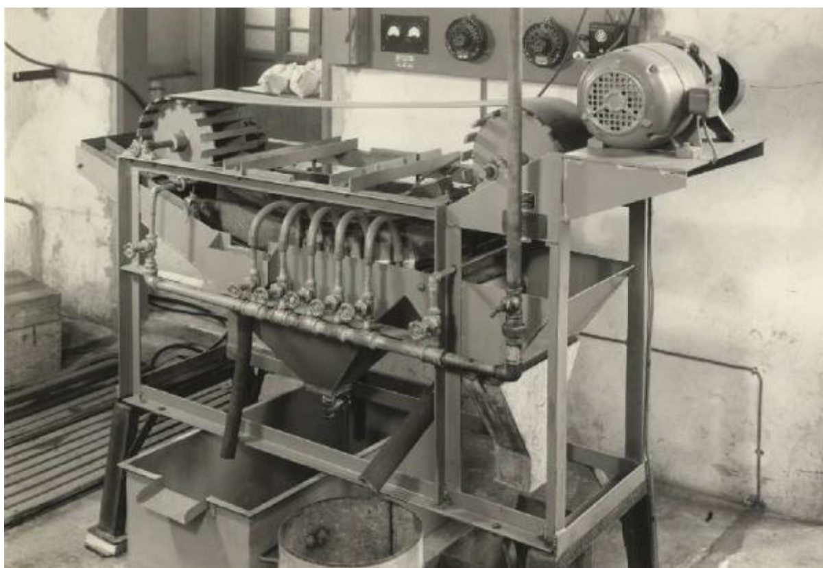
SEPARATORE MAGNETICO - MAGNETIC SEPARATOR
