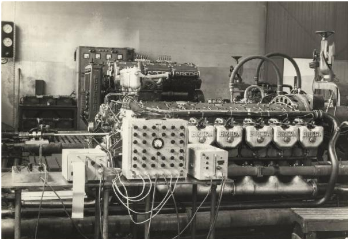
ANALISI SOLLECITAZIONI DINAMICHE - DYNAMIC STRESS ANALYSIS
