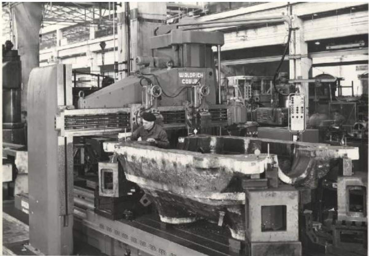
Piatta Waldrich-Coburg a corando oleodinamico - Tavola 4000x2000 - Altezza piattabile 1600 - Portata In lavorazione: corpo inferiore esterno A.P. per turbina a vapore
