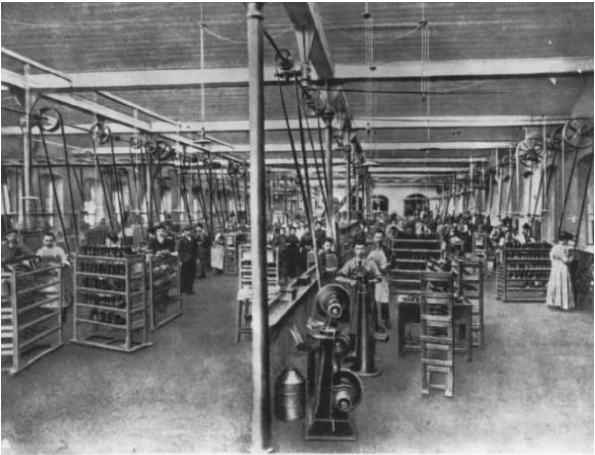
VEDUTA GENERALE DEL SALONE MACCHINE.
